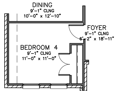
* Bedroom 4 in lieu of Study Option First Floor Plan
