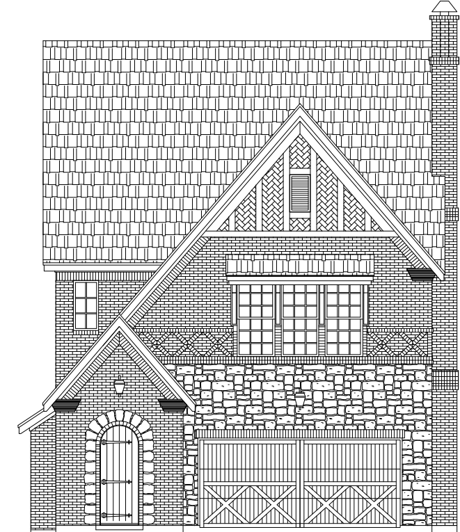
Elevation A
