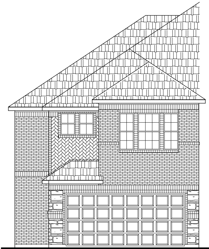
Elevation A
