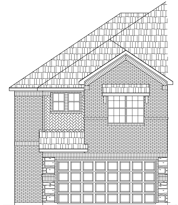
Elevation B
