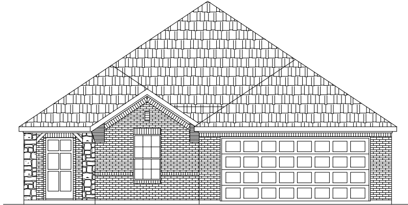
Elevation A
