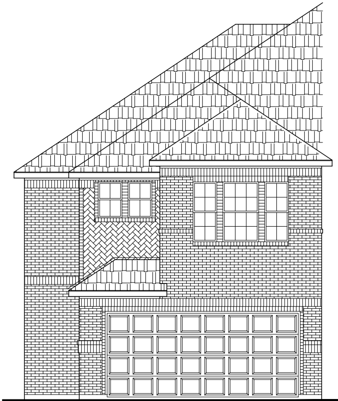
Elevation A
