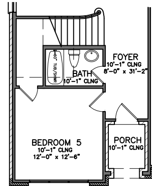
* Bedroom 5 in lieu of Study Option First Floor Plan
